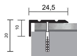
Pravouhý schodový profil, hliník
