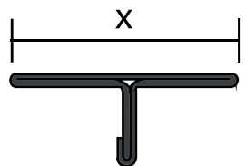
Přechodový T profil, nerezová ocel
