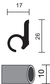
Schodový ukončovací profil pro laminátové podlahy, hliník
