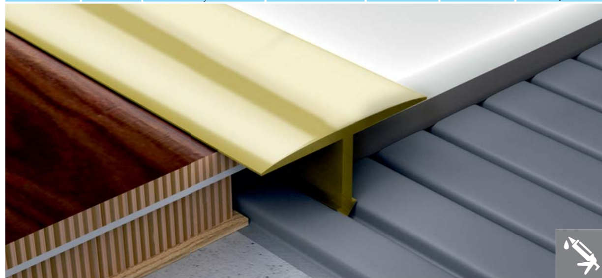
Ukončovací profil, hliník
