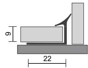
Pravouhý profil, mosaz
