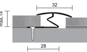
Přechodový profil Z-et, hliník
