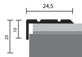
Pravouhý schodový profil samolepící, hliník
