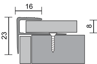
Schodový ukončovací profil pro laminátové podlahy, hliník
