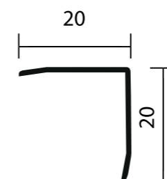
Ochranný pravouhý profil, nerezová ocel
