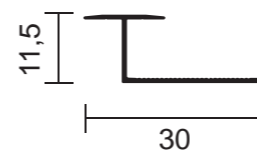
Ohebný T profil, hliník
