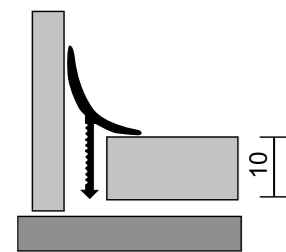
Rohový profil zadní, hliník
