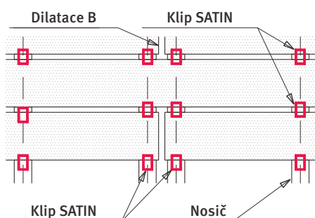
Obr. 5 Napojování terasových prken pomocí rovnoběžných nosičů
