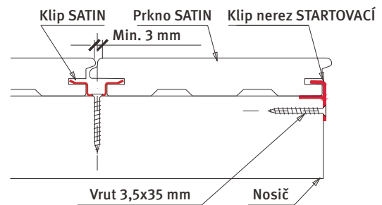
Obr. 3 Kotvení terasových prken SATIN pomocí nerezových klipů a vrutů
