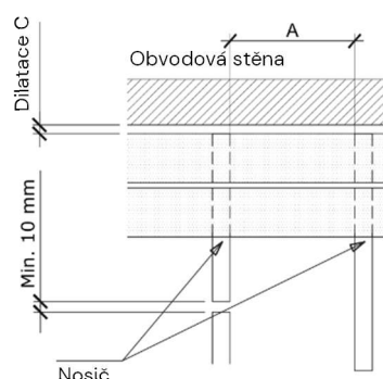
Obr. 2 Pokládka nosičů a vzdálenost mezi nimi
