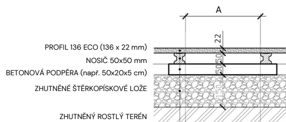
Obr. 1 Skladba terasy při použití nosičů GRANDECK® 50x50 mm
