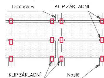
Obr. 5 Napojování terasových prken pomocí KLIPU ZÁKLADNÍ
