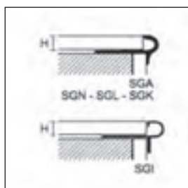
SGK/11 pochromovaná mosaz
