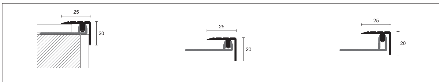
G/1/SF hliník potažen Alcrom® Plus
