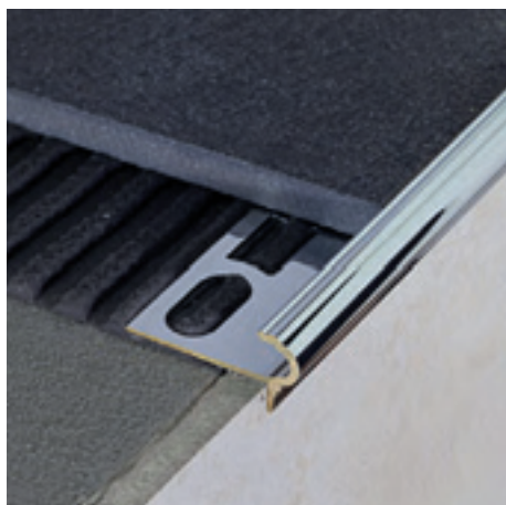
SGK/11 pochromovaná mosaz
