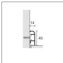
97/4TMSF lesklý hliník broušený titan
