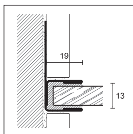
GPS2/19 nerez ocel broušená AISI 304 DIN 1.4301
