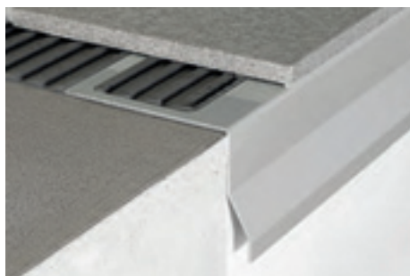
CPBV/55 lakovaný hliník šedý popel RAL 7038
