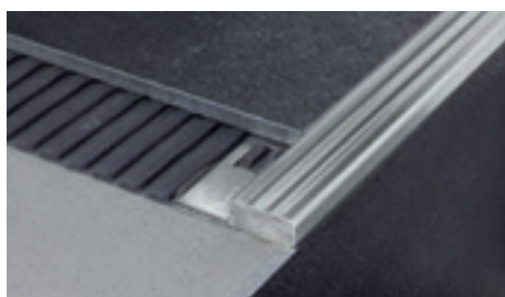
SIS/10 nerez ocel broušená AISI 304 - DIN 1.4301
