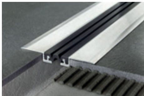
GJF/40 hliník přírodní + EPDM černá
