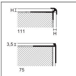
111/4/F eloxovaný hliník stříbro
