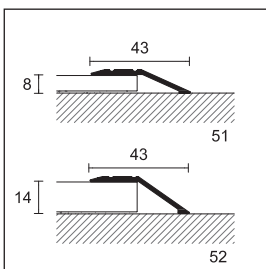
51/A eloxovaný hliník zlato
