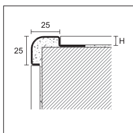
IL/10 nerez ocel leštěná AISI 304 DIN 1.4301
