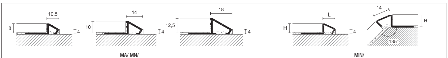
MIN/10 nerez ocel leštěná AISI 304 DIN 1.4301
