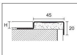
SIX/10 nerez ocel broušená AISI 304 - DIN 1.4301 + protisklizový černý 25 mm
