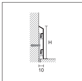
95/7 eloxovaný hliník stříbro
