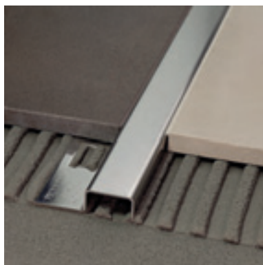
UI/10 nerez ocel AISI 304 DIN 1.4301
