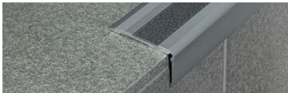
76/F eloxovaný hliník stříbro + protiskuzový černý
