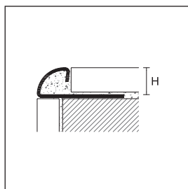
RKN/10 pochromovaná mosaz
