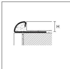
RI/10 nerez ocel AISI 304 DIN 1.4301
