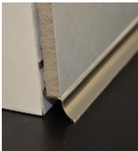
PIN/10 nerez ocel AISI 304 DIN 1.4301
