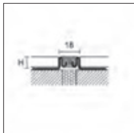
NI/ nerez ocel AISI 304 - DIN 1.4301 + černá guma
