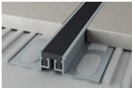
NA/10 hliník přírodní + černá guma
