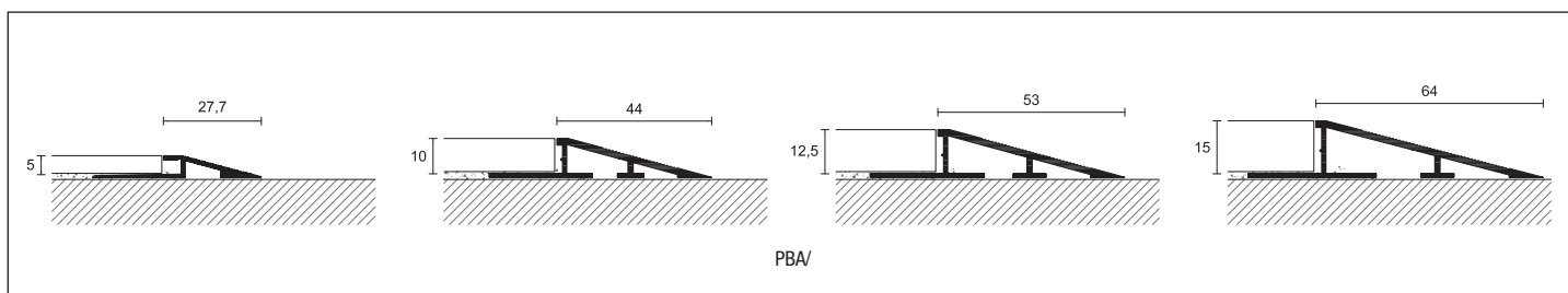
PBA/10 eloxovaný hliník stříbro
