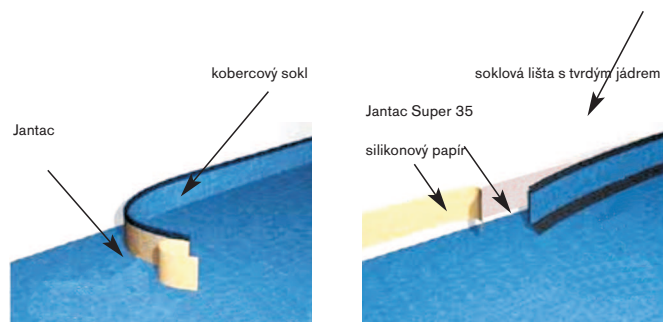
Montáž kobercových soklů s páskou Jantac
