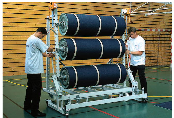
Zavěšení role na stojan s pomocí transportního a odvíjecího zařízení
