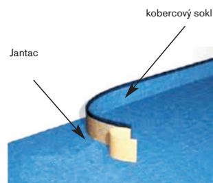
Montáž kobercových soklů s páskou Jantac
