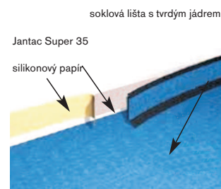
Montáž soklových lišt s tvrdým jádrem s páskou Jantac Super 35
